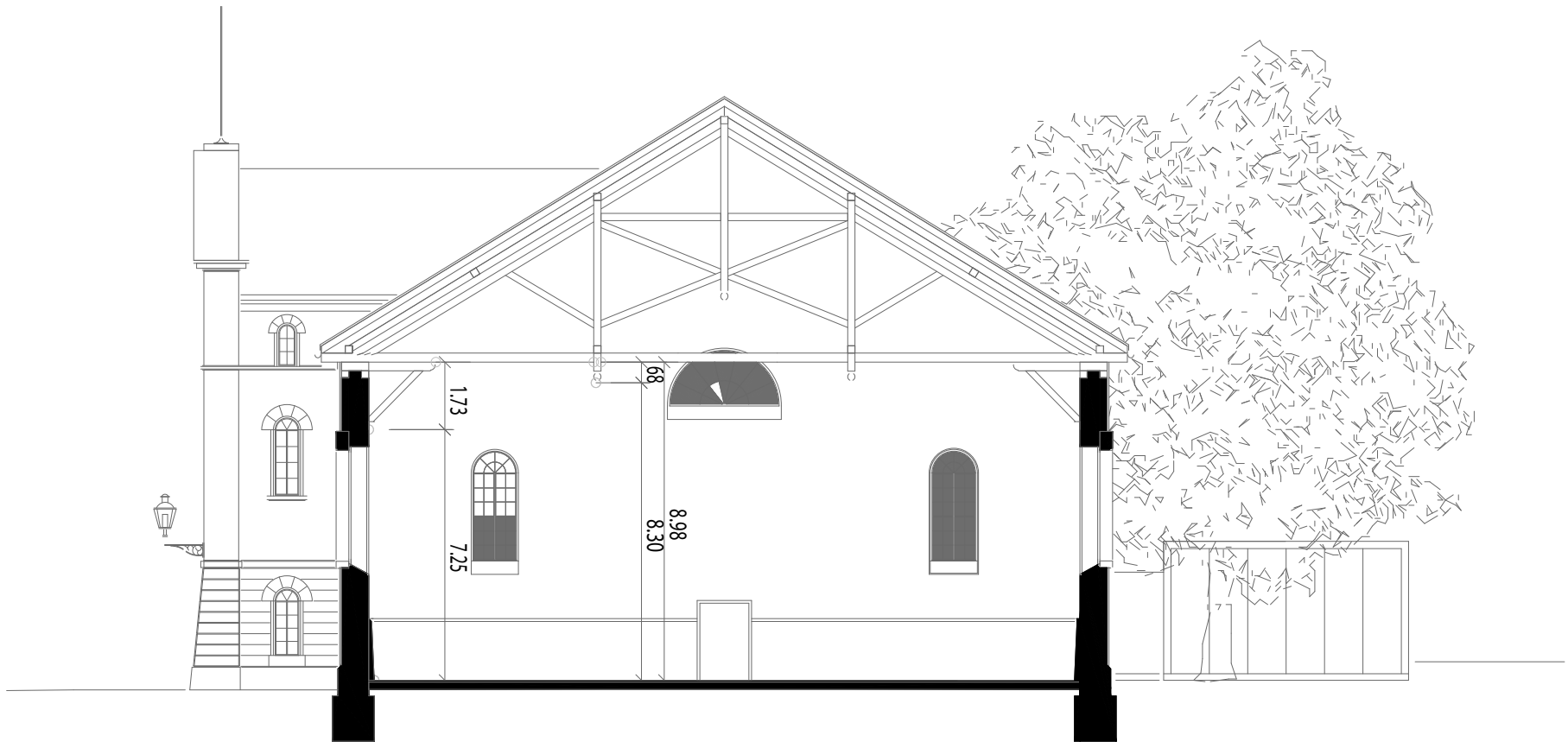
Querschnitt
